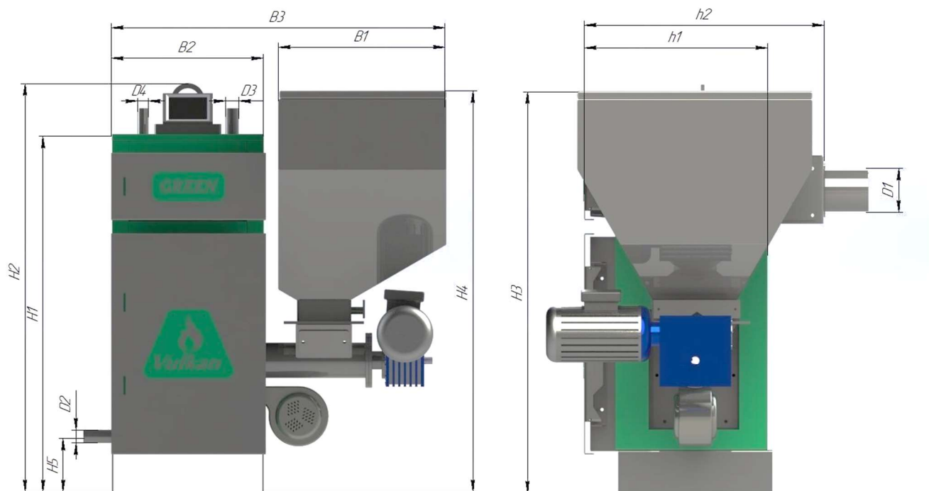
Рисунок 1. Габаритные размеры GREEN
