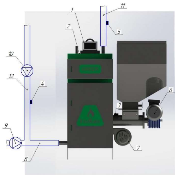
Рисунок 9 — Схема подключения блока управления к котлу. 1-контроллер (подключается к сети 220В); 2-датчик системы отопления (устанавливается в гильзу); 3-датчик шнека; 4-датчик горячего водоснабжения (ГВС); 5-аварийный датчик (термик); 6-мотор-редуктор; 7-вентилятор; 8-труба обратной линии от отопления; 9-насос системы отопления; 10-насос ГВС; 11-труба подачи; 12-труба обратной линии от бойлера ГВС.
