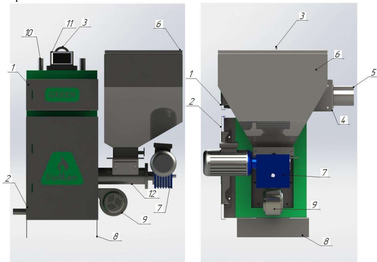
Рисунок 3 — Схема размещения составных элементов в котлах серии GREEN. 1- дверца теплообменника; 2-дверца топочной камеры и зольника; 3-ухо транспортное; 4-короб дымохода; 5-труба дымовая; 6-бункер топлива; 7-мотор-редуктор; 8- опора котла; 9-вентилятор наддува; 10- патрубок под группу безопасности; 11-контроллер; 12-труба топливоподачи
